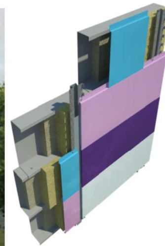
Beispiel: Glattblechfassade
